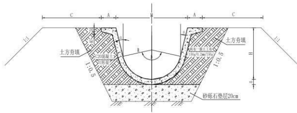
U形渠道断面图
