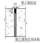
伸缩缝详图 1:10
