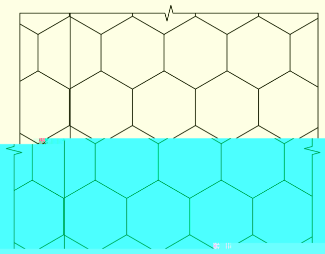
预制块排列布置图
