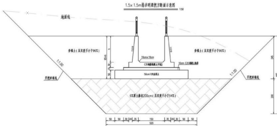
1.5×1.5m 排洪明渠挖方断面示意图
